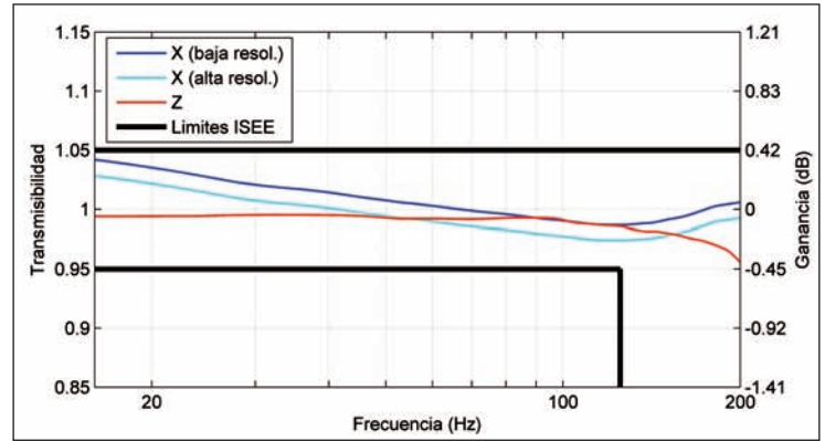
[Figura 4].- Transmisibilidad de los sismógrafos.
