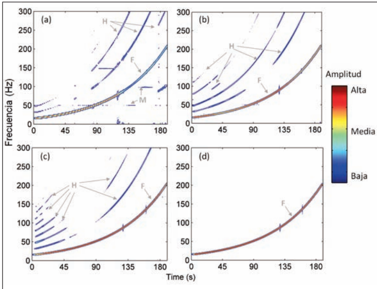
[Fig. 3].- Espectrogramas para el sismógrafo Z: colocado libremente a baja velocidad, LB (a), sujeto con saco con arena a baja velocidad, SB (b) y alta velocidad, SA (c), y anclado a alta velocidad, AA (d).
