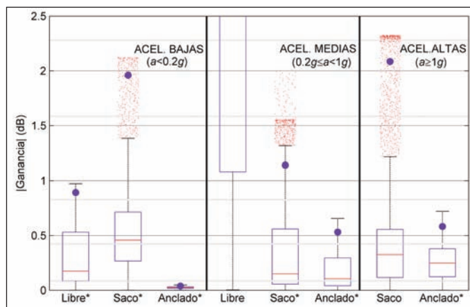
[Figura 7] .- Distribuciones del valor absoluto de la ganancia debida al acoplamiento para diferentes niveles de aceleración.
